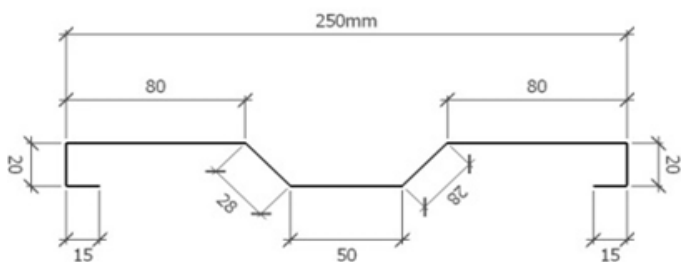
Элемент ограждения
